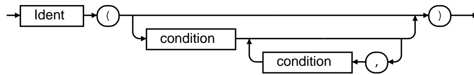
call:
