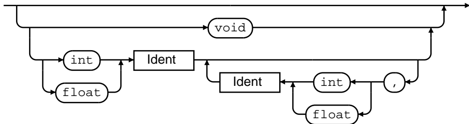
parameters:
