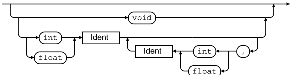
parameters:
