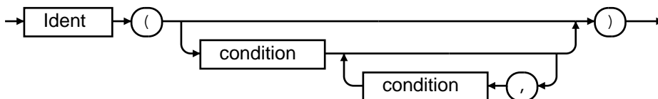
call:
